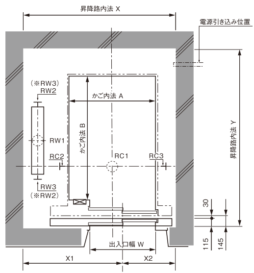
昇降路平面図
